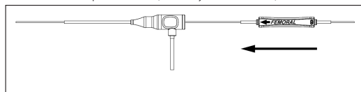
Obrázek 11: Zavedení kazety do ústí sheathu po vodícím drátu (zobrazena je femorální varianta)
