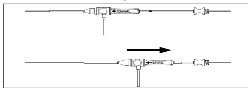
Kuva 12: Suodatimen vapauttaminen ohjainlanka pitkin paljastusmenetelmää käyttäen (kuvassa reidessä käytettävä suunta)
