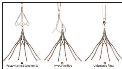
Slika 13: Vadenje filtra
