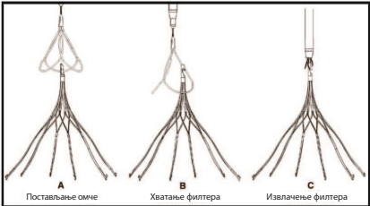
Слика 13: Вађење филтера
