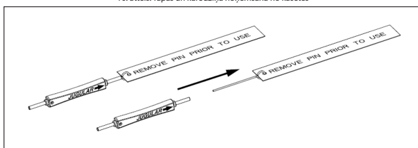
10. attēls. Tapas un karodziņa noņemšana no kasetes
