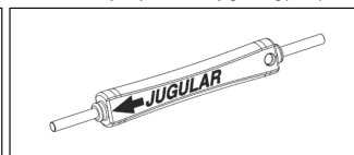
Slika 5B: Usmjerenje uložka kod jugularnog pristupa
