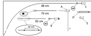
Фигура 1: Филтърна система Option™ ELITE
